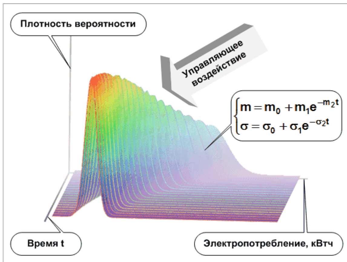
Рис. 4.14. Изменение формы нормального распределения при модельной реализации управляющего воздействия
